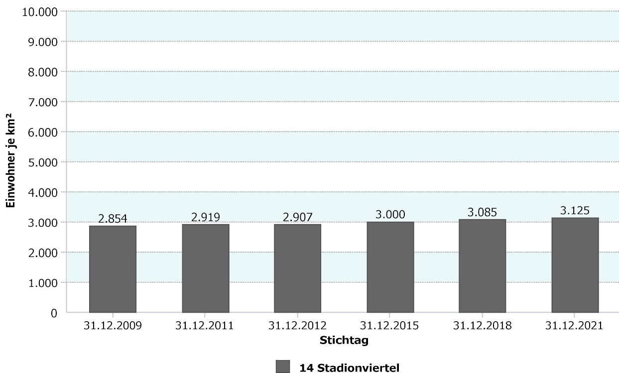
Entwicklung Einwohnerdichte
